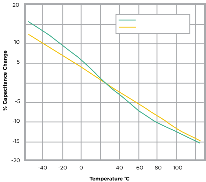
C-200/C-400
